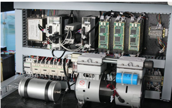
全轴采用松下伺服系统+进口真空泵+负压存储器
