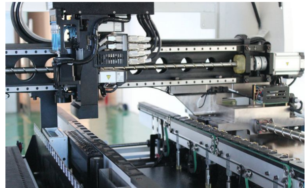
高精度 NSK 丝杆+导轨系统
